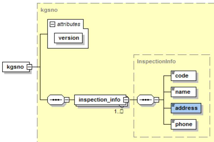
Рисунок Схема файла справочника KGSNO.
