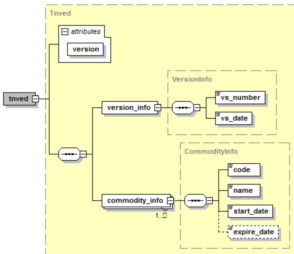
Рисунок 5.10.1. Схема файла справочника ТН ВЭД.
