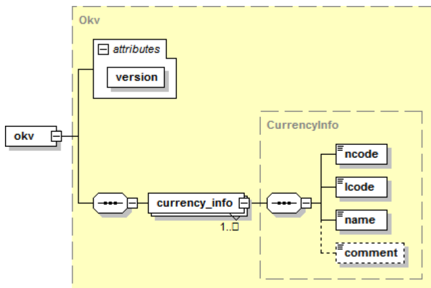
Рисунок 5.8.1. Схема файла справочника ОКВ.
