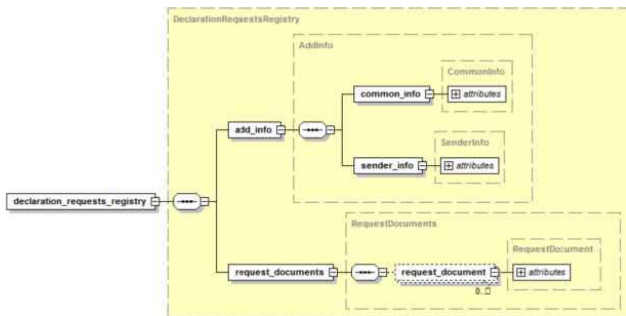
Рисунок 3.3.1 Схема файла реестра запросов.
