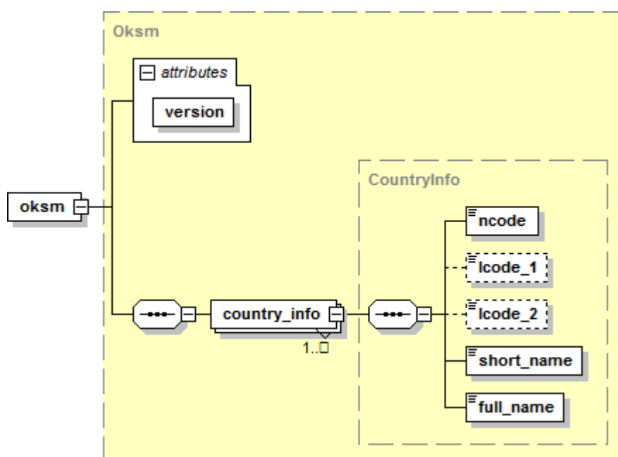
Рисунок 5.5.1. Схема файла справочника ОКСМ.
