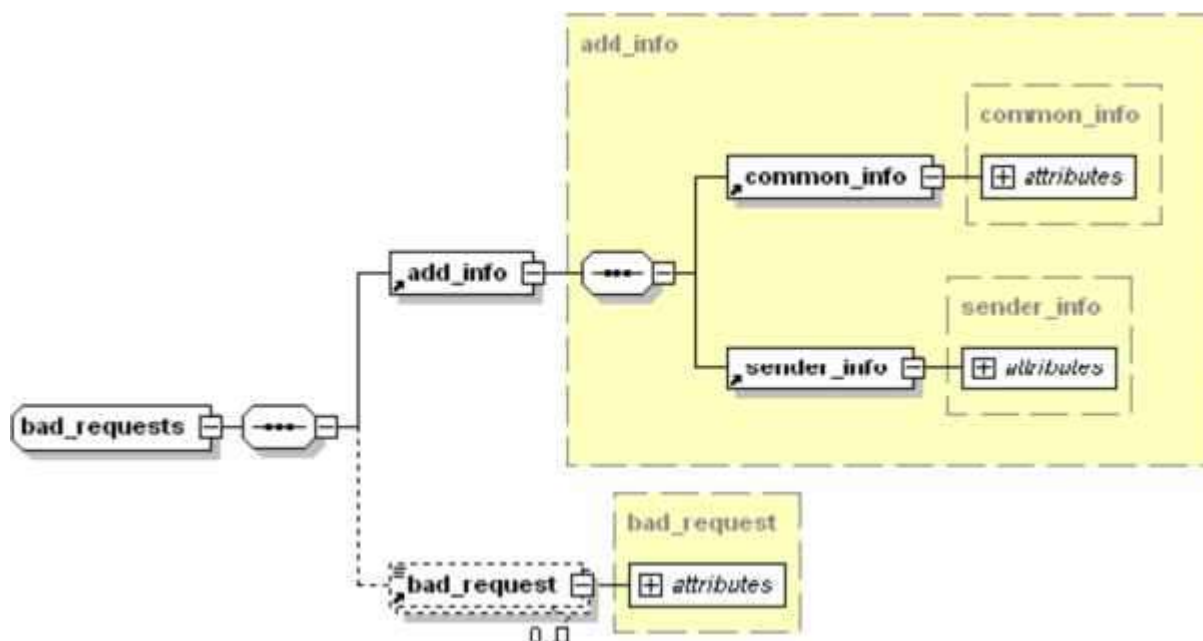
Рисунок 4.3.1 Схема файла реестра уведомлений.
