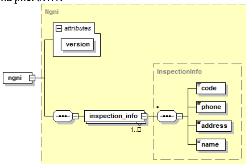
Рисунок 5.1.1. Схема файла справочника NGNI.
