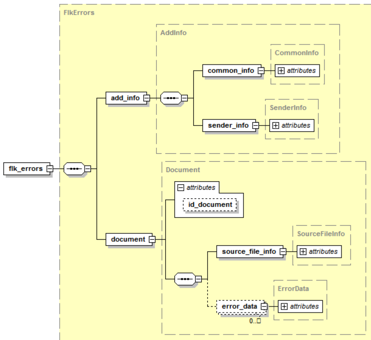
Рисунок 6.3.1 Схема файла протокола ФЛК.
