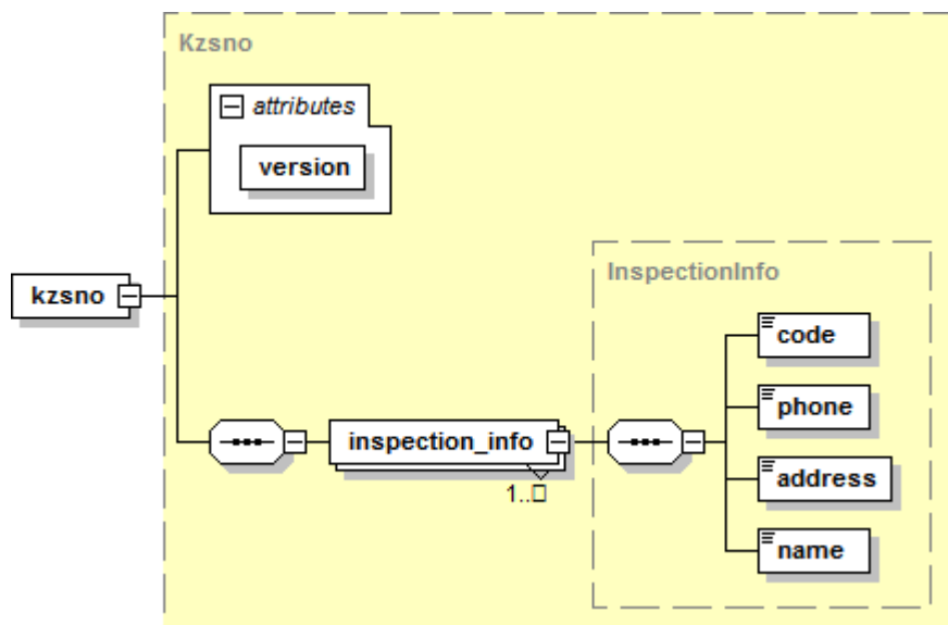
Рисунок 5.2.1. Схема файла справочника KZSNO.
