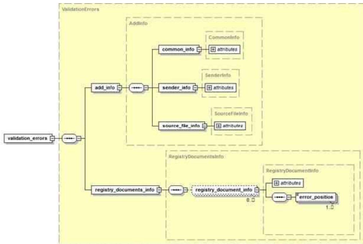
Рисунок 7.3.1 Схема файла протокола идентификации.
