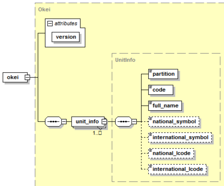
Рисунок 5.7.1. Схема файла справочника ОКЕИ.
